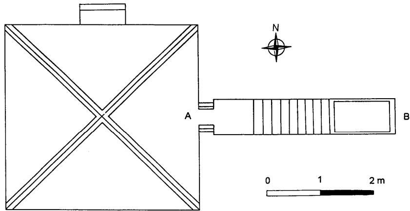
Fig. 1 : Plan de la crypte
